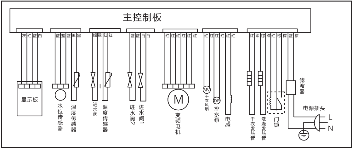
电气原理图
